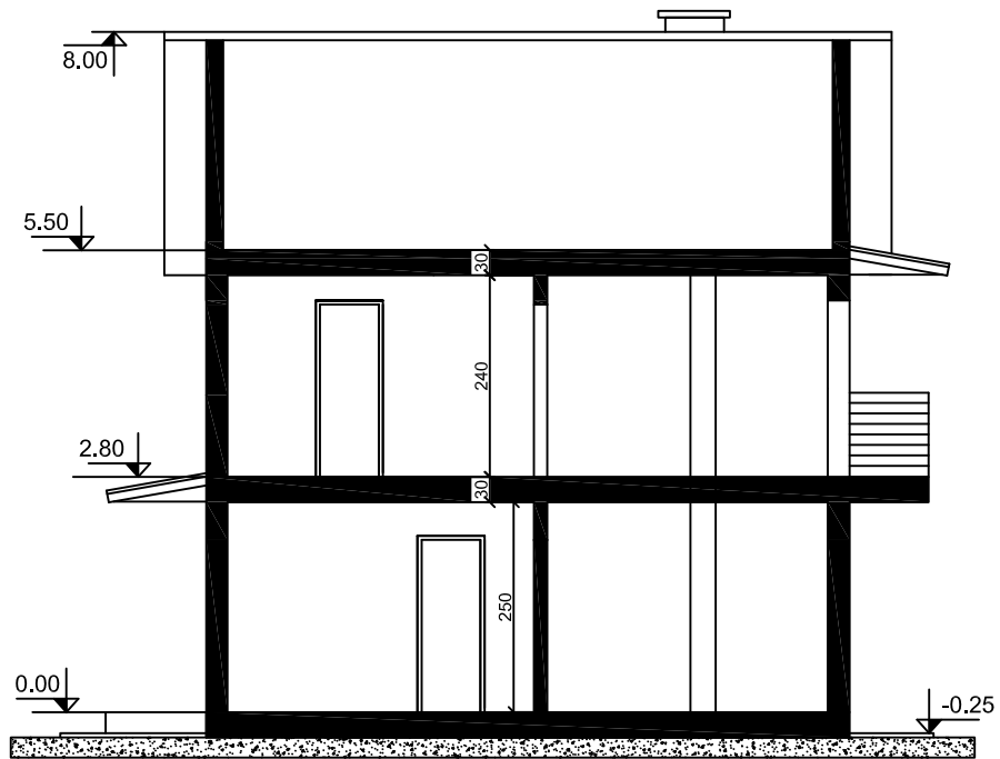
Sectione A-A
