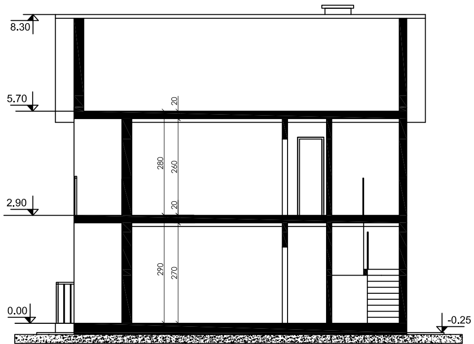
Sectiune A-A
