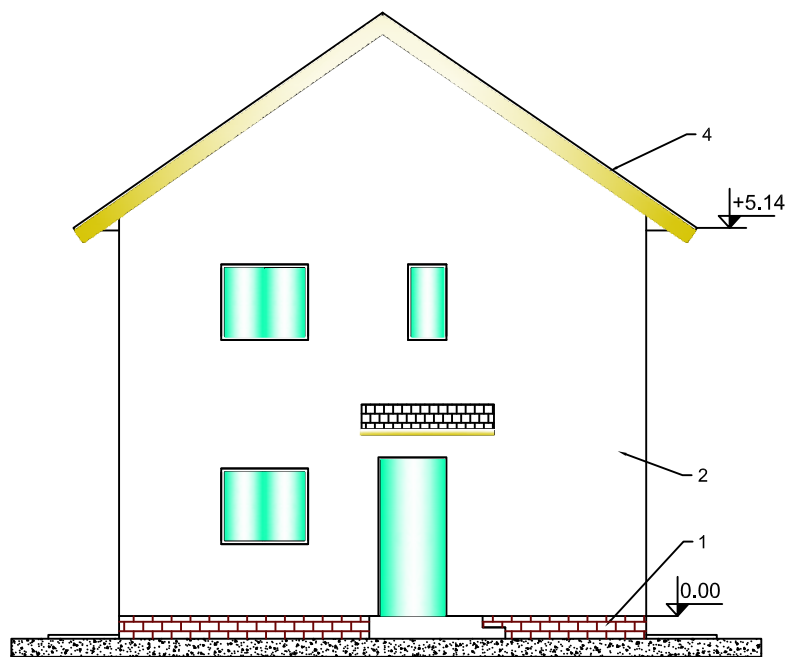
Fatada Nord
