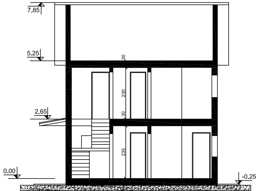
Sectiune A-A
